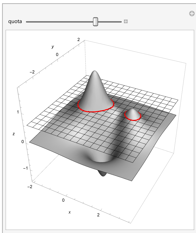
Visualizzazione di un gruppo di linee di livello
